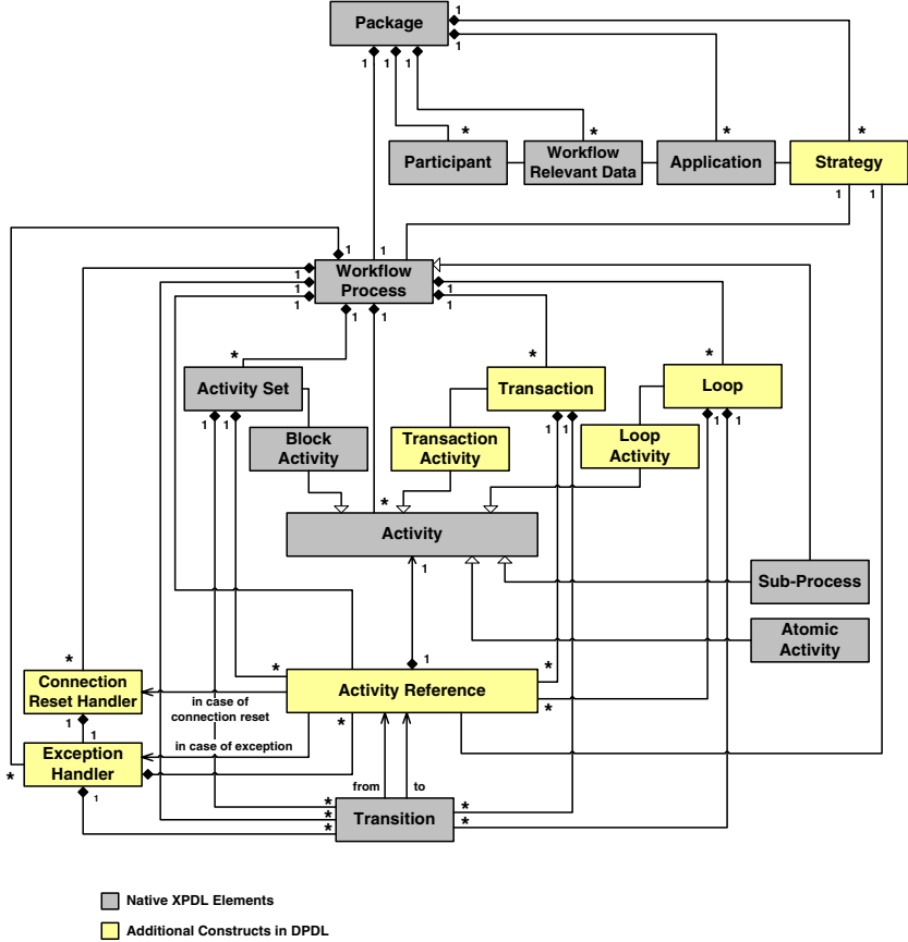
Fig. 2. DPDL Meta-model
